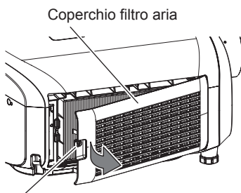
Vite di fissaggio del coperchio filtro aria
