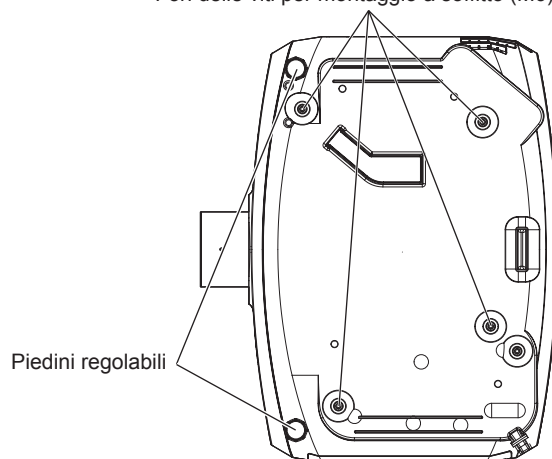
La posizione dei fori delle viti per il montaggio a soffitto e dei piedini regolabili
