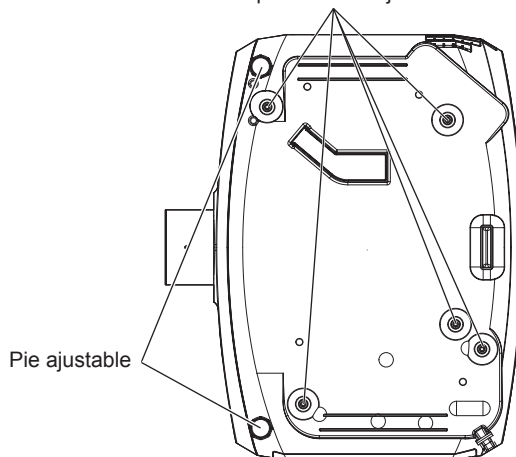
Posiciones de los orificios de tornillo para el montaje en el techo y uso de pie ajustable
