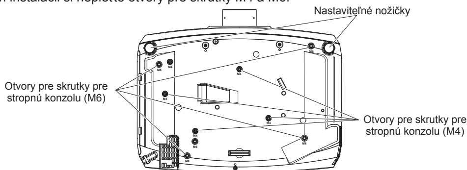
Polohy otvorov pre skrutky pre stropnú konzolu a pre nastaviteľné nožičky.
