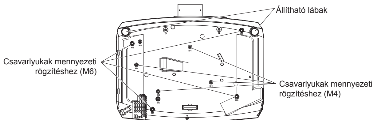
A mennyezeti rögzítésre szolgáló csavarlyukak és állítható lábak helyei
