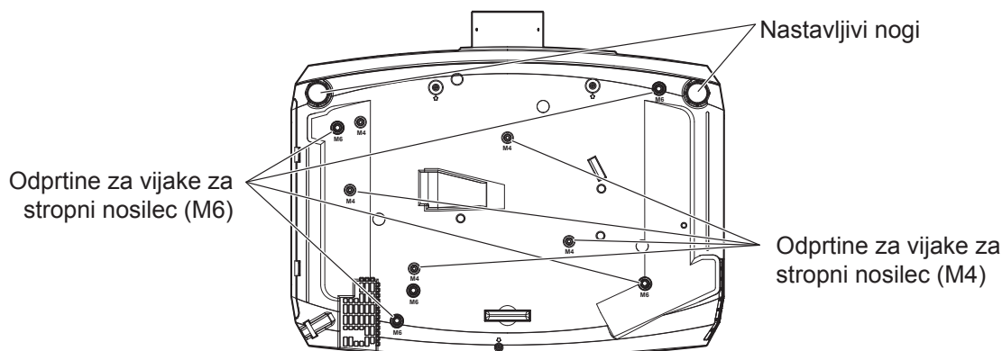
Položaj odprtín za vijake za stropni nosilec in nastavljivih nog
