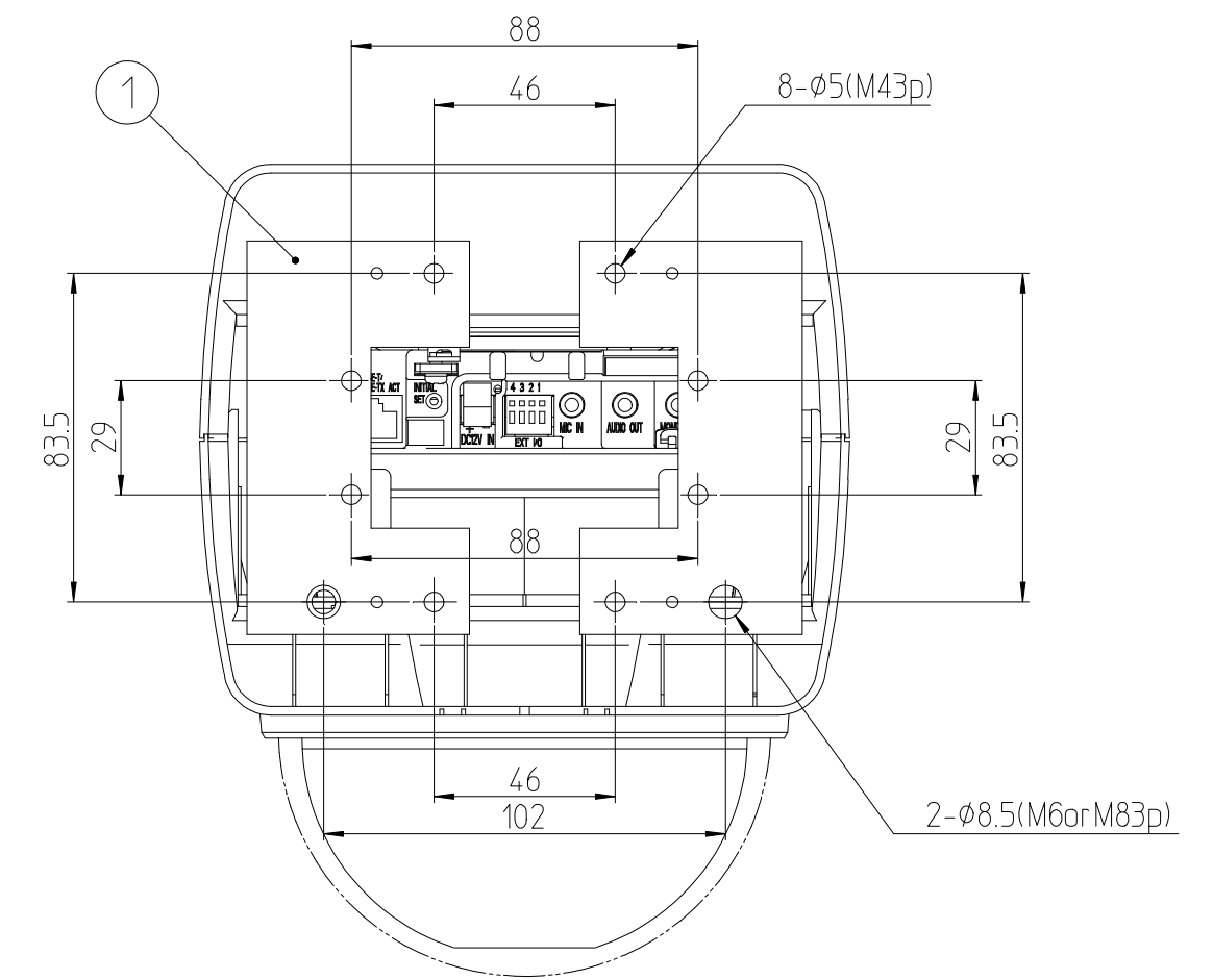
A-A 断2°□
