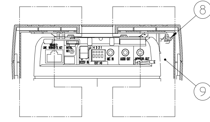
A-A 断2°□
