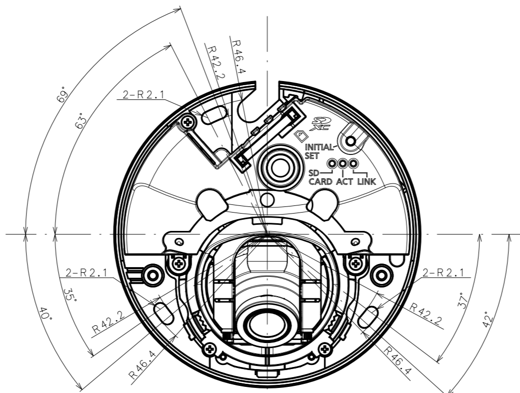
カメラ取付寸法 Mounting dimensions of camera
