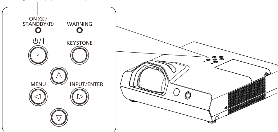
Betriebsanzeige <ON(G)/STANDBY(R)>
