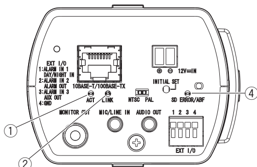
<Vue arrière>
