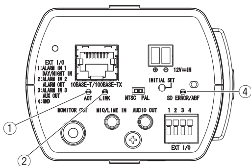
<Вид сзади>
