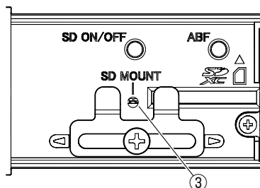
<Face intérieure de couvercle coulissant latéral>
