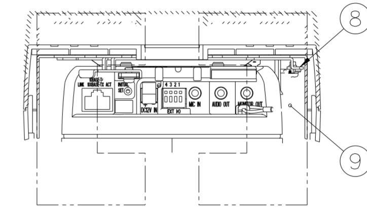
A-A 断面図
