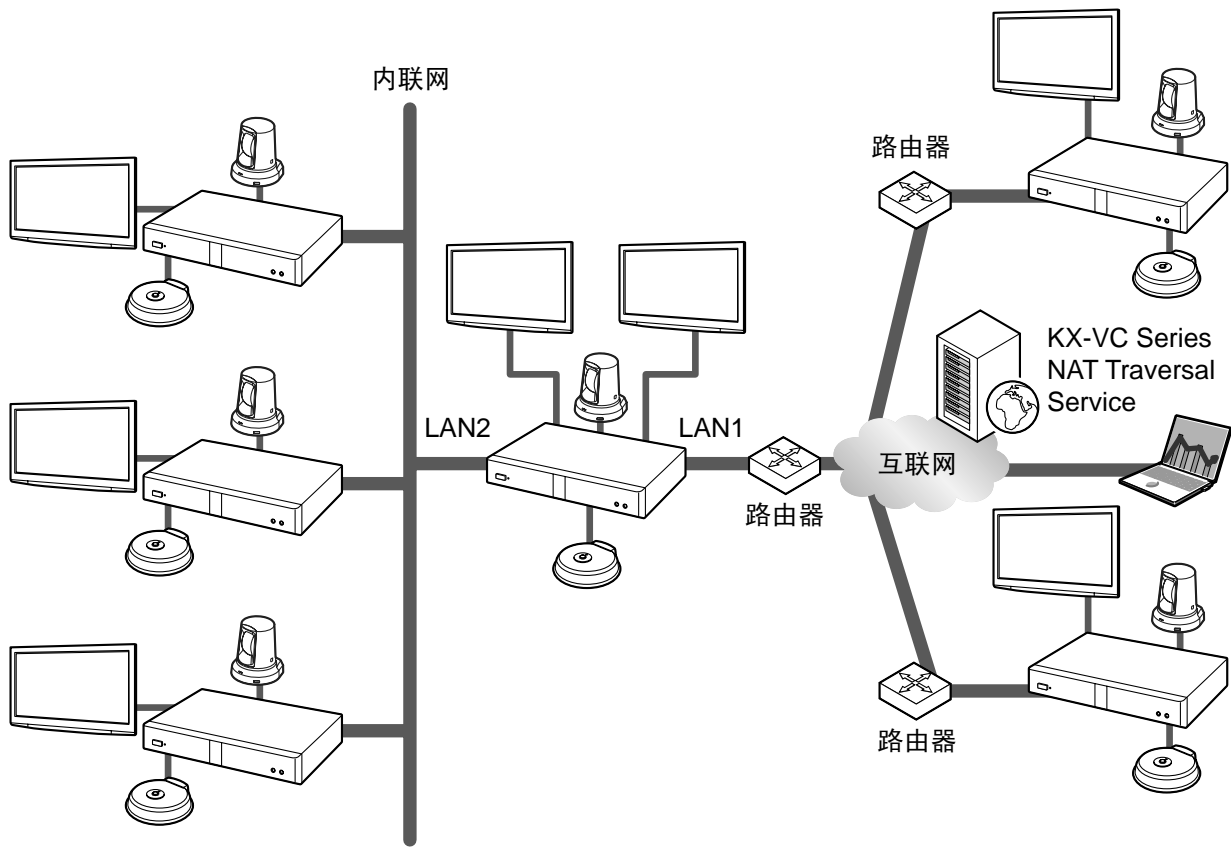
图（使用内联网/KX-VC Series NAT Traversal Service时） 兼容LAN1和LAN2 (KX-VC1600、KX-VC2000)
