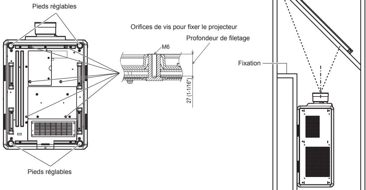
Positions des orifices de vis pour fixer le projecteur et les pieds réglables
